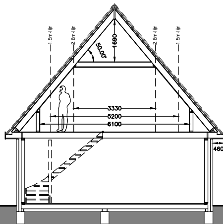
DOORSNEDE
